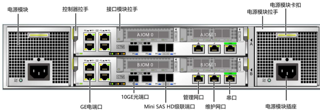
图1-5 控制框后视图
