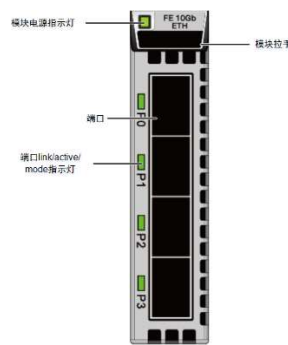
图1-50 速率为 10Gbit/s 的 TFCQ IO 接口模块
