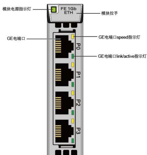
图1-43 GE 电接口模块
