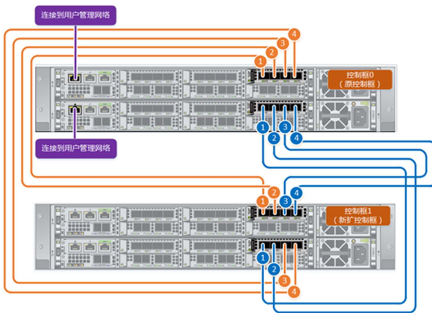
图1-70 图示：RDMA ScaleOut 4 控直连组网
