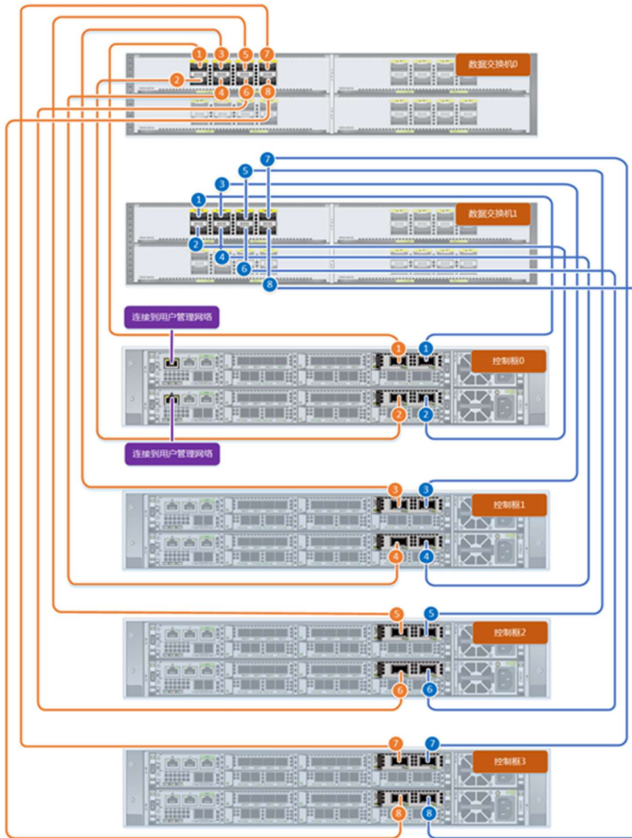
图1-71 图示：RDMA ScaleOut 8 控交换组网
