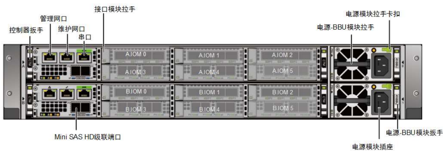
图1-32 控制框后视图（板载 100Gb RDMA 端口）
