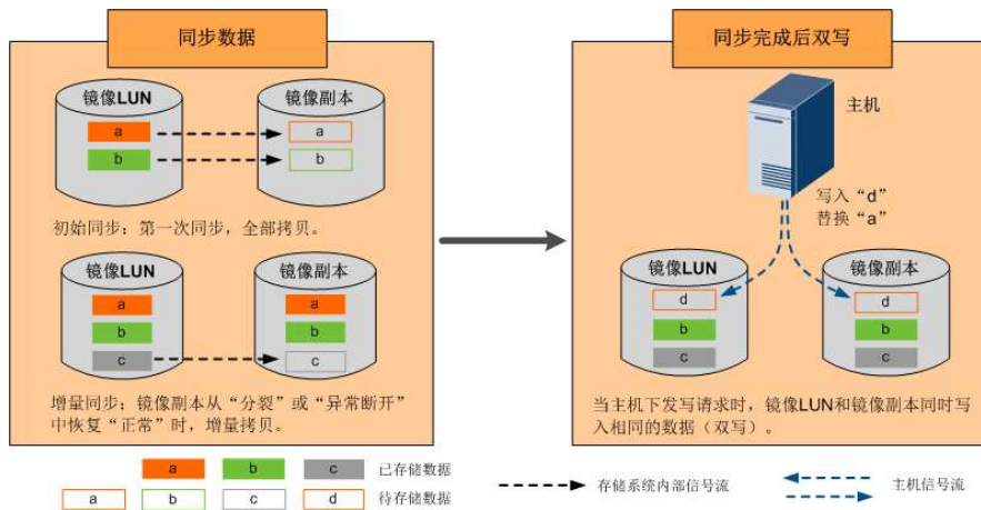
图1-98 卷镜像同步过程
