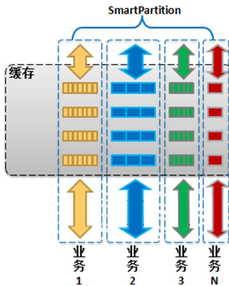
图1-83 缓存分区示意图
