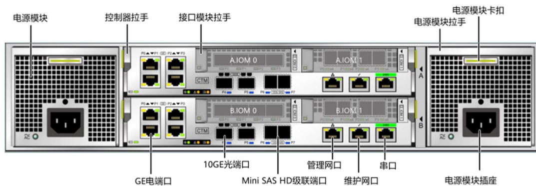
图1-13 控制框后面板指示灯
