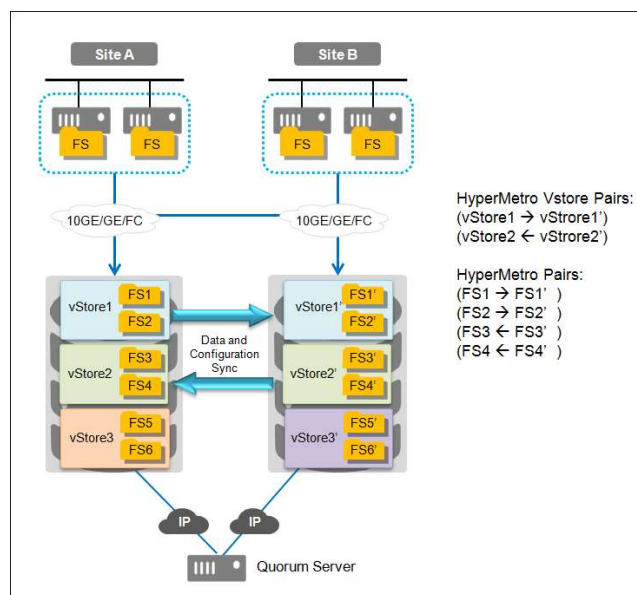
图1-95 基于 vStore 的 HyperMetro 架构
