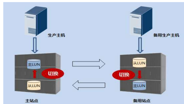
图1-89 同步复制主从切换示意图
