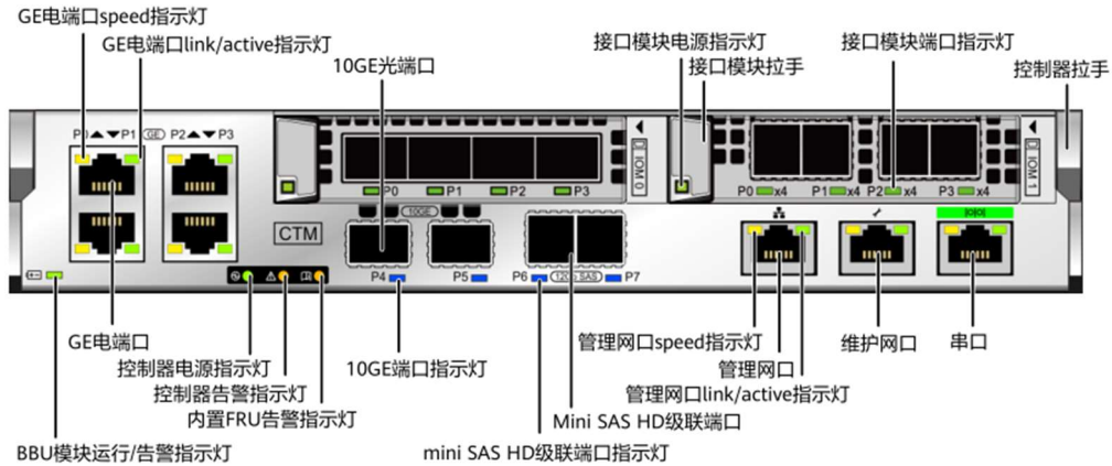
图1-7 控制器接口信息
