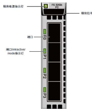
图1-53 速率为 32Gbit/s 的 TFCQ IO 接口模块
