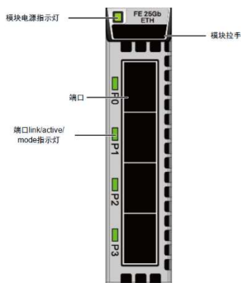
图1-52 速率为 25Gbit/s 的 TFCQ IO 接口模块
