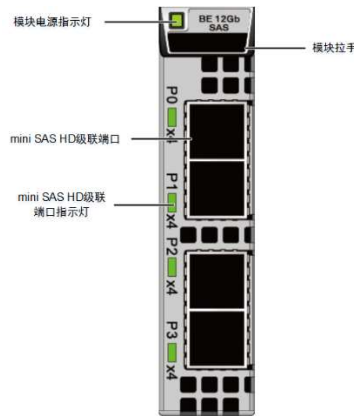
图1-54 12Gb SAS 级联模块
