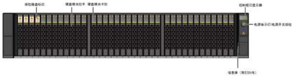
图1-30 2U 36 盘位控制框前视图
