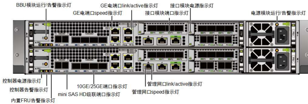
图1-26 控制框后面板指示灯
