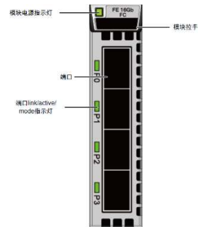
图1-51 速率为 16Gbit/s 的 TFCQ IO 接口模块
