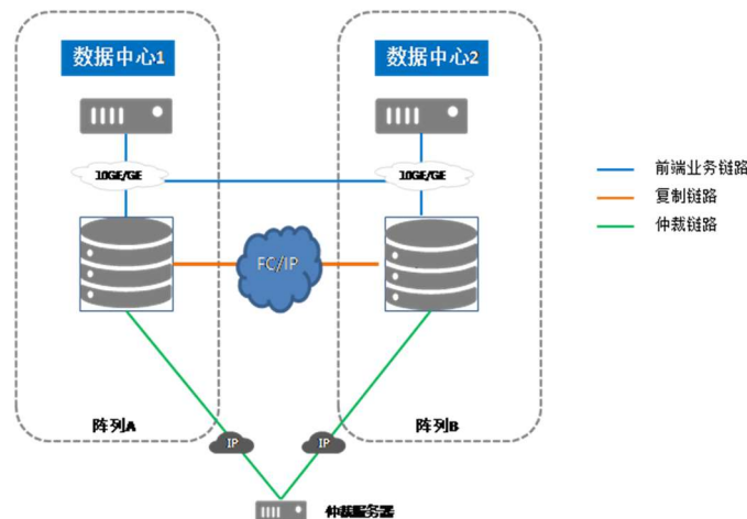
图1-94 NAS 双活逻辑组网图
