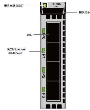
图1-49 速率为 8Gbit/s 的 TFCQ IO 接口模块
