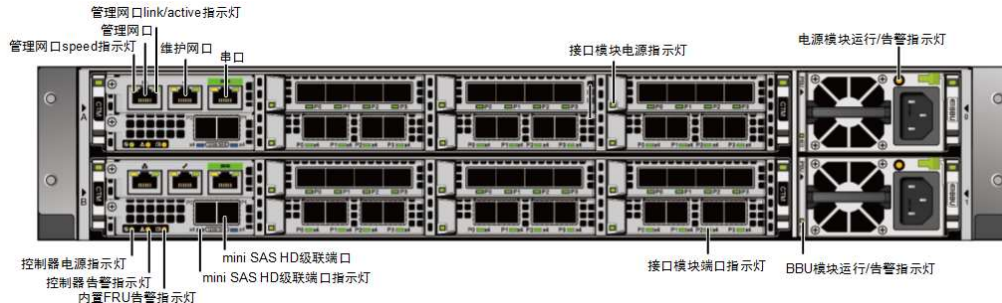
图1-42 控制框后面板指示灯
