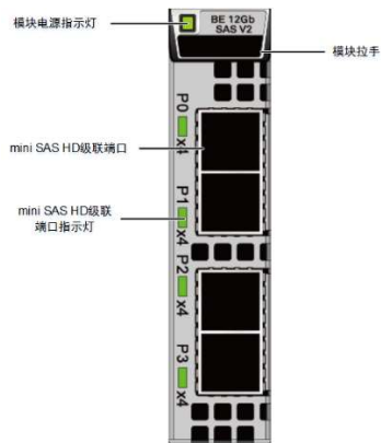
图1-55 12Gb SAS V2 共享级联模块
