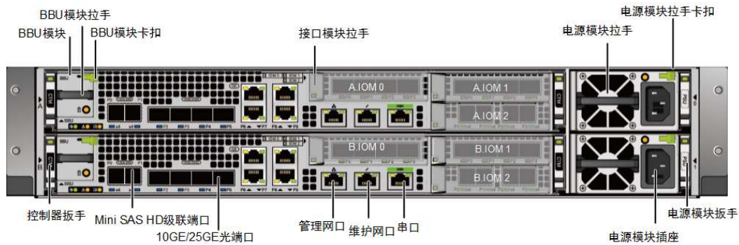
图1-16 控制框后视图
