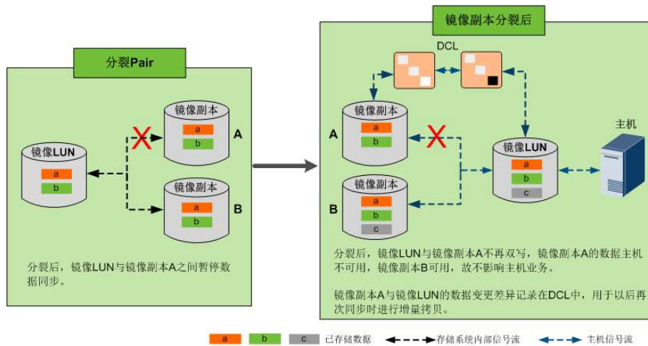
图1-99 卷镜像分裂过程
