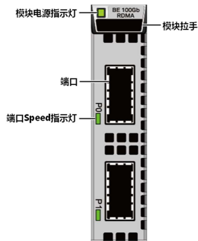
图1-48 BE 100Gb RDMA 接口模块
