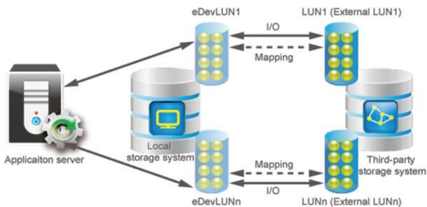
图1-75 异构虚拟化技术示意图
