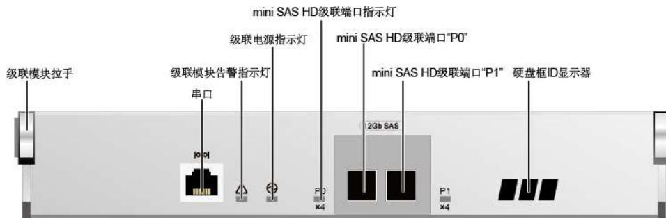
图1-63 级联模块接口信息
