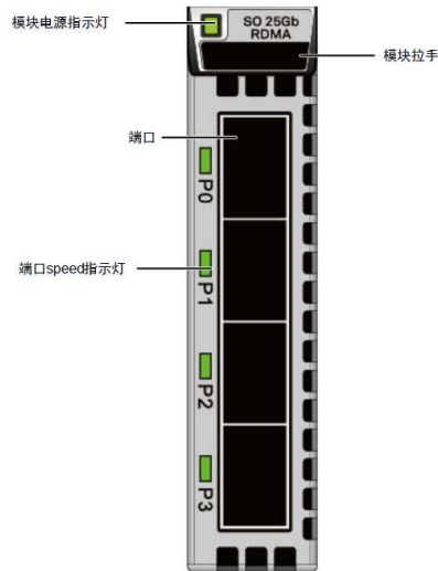
图1-44 25Gb RDMA 接口模块
