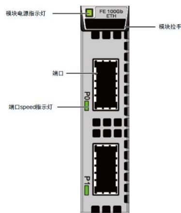
图1-46 100GE 接口模块
