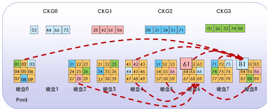
图1-74 RAID2.0+快速重构示意图（二）
