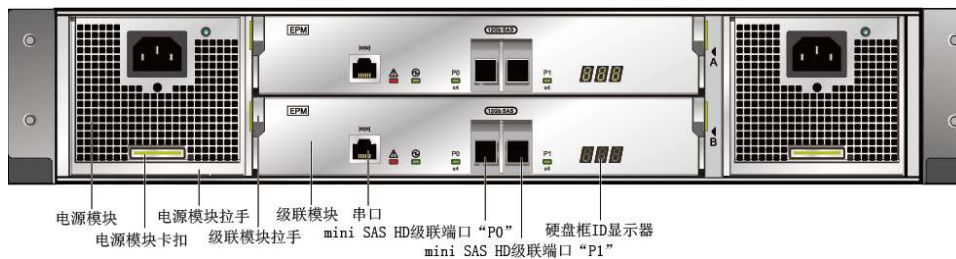
图1-59 硬盘框后视图
