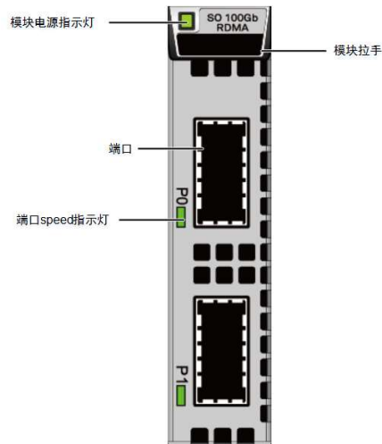
图1-47 SO 100Gb RDMA 接口模块
