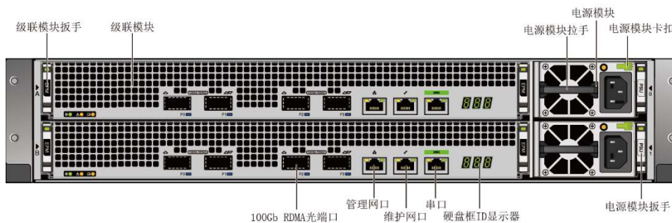
图1-60 配置交流电源模块硬盘框后视图
