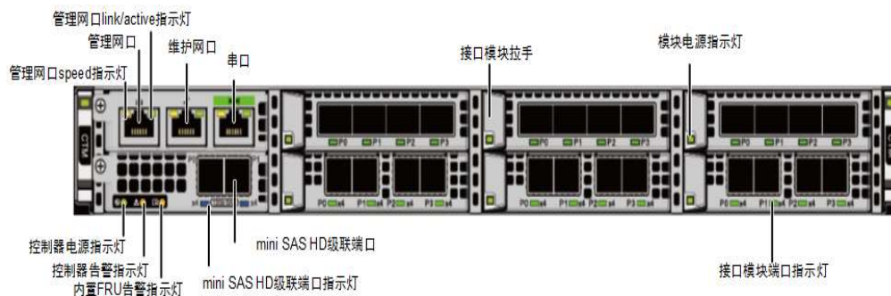
图1-35 控制器接口信息
