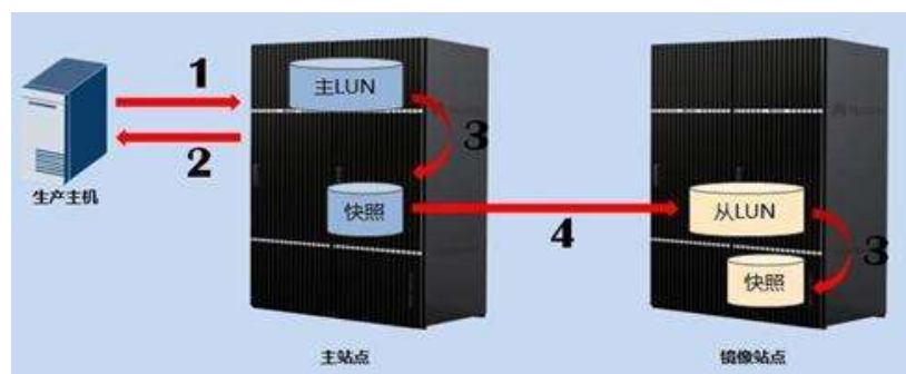
图1-91 异步复制技术原理示意图
