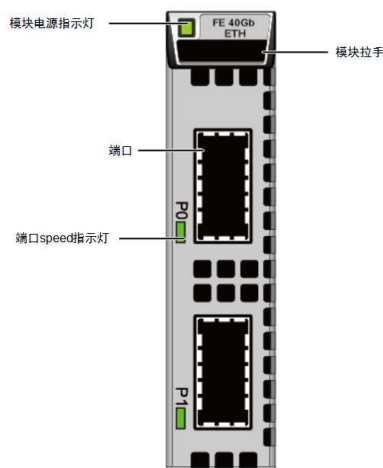
图1-45 40GE 接口模块
