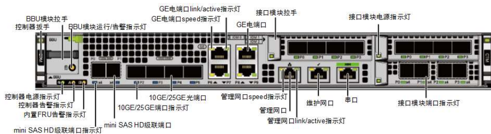
图1-19 控制器接口信息
