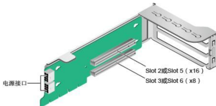
图 4.10: 1x8+1x16 Riser 卡
