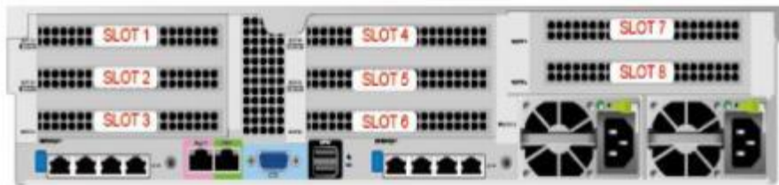
图 4.15: PCIe 插槽
