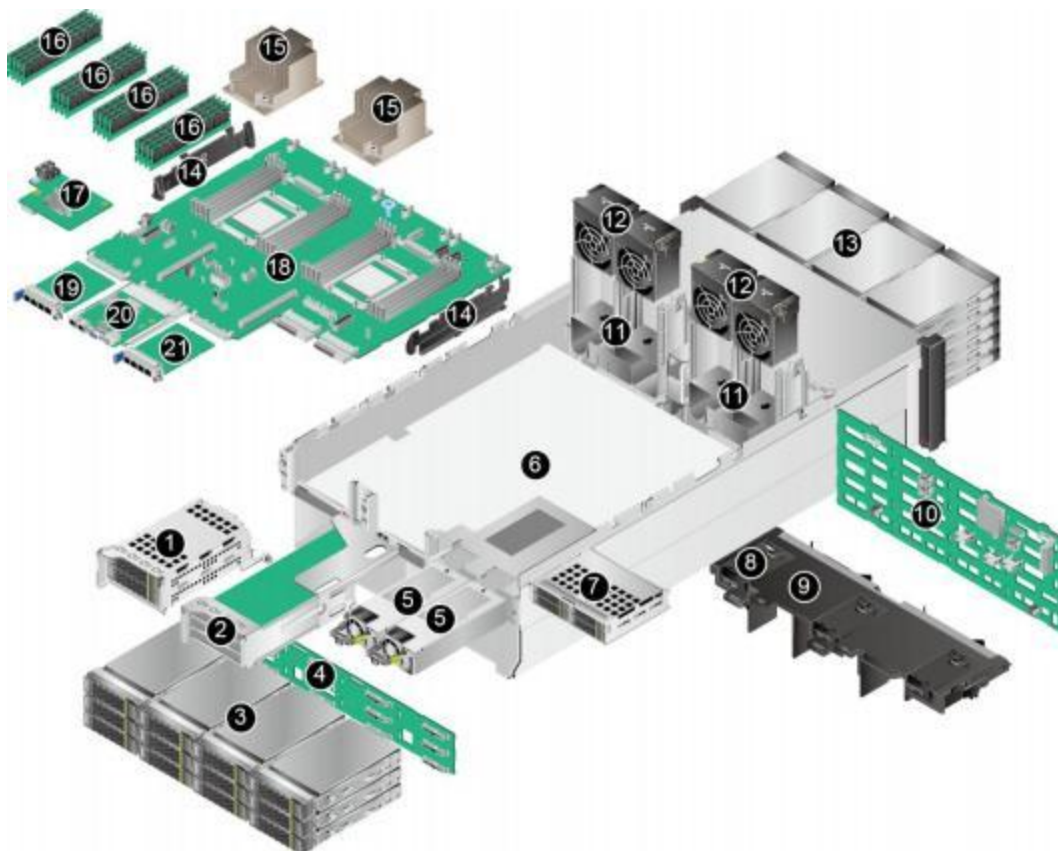
图 4.17：物理结构（配置鲲鹏 920 5220 或 3210 处理器）
