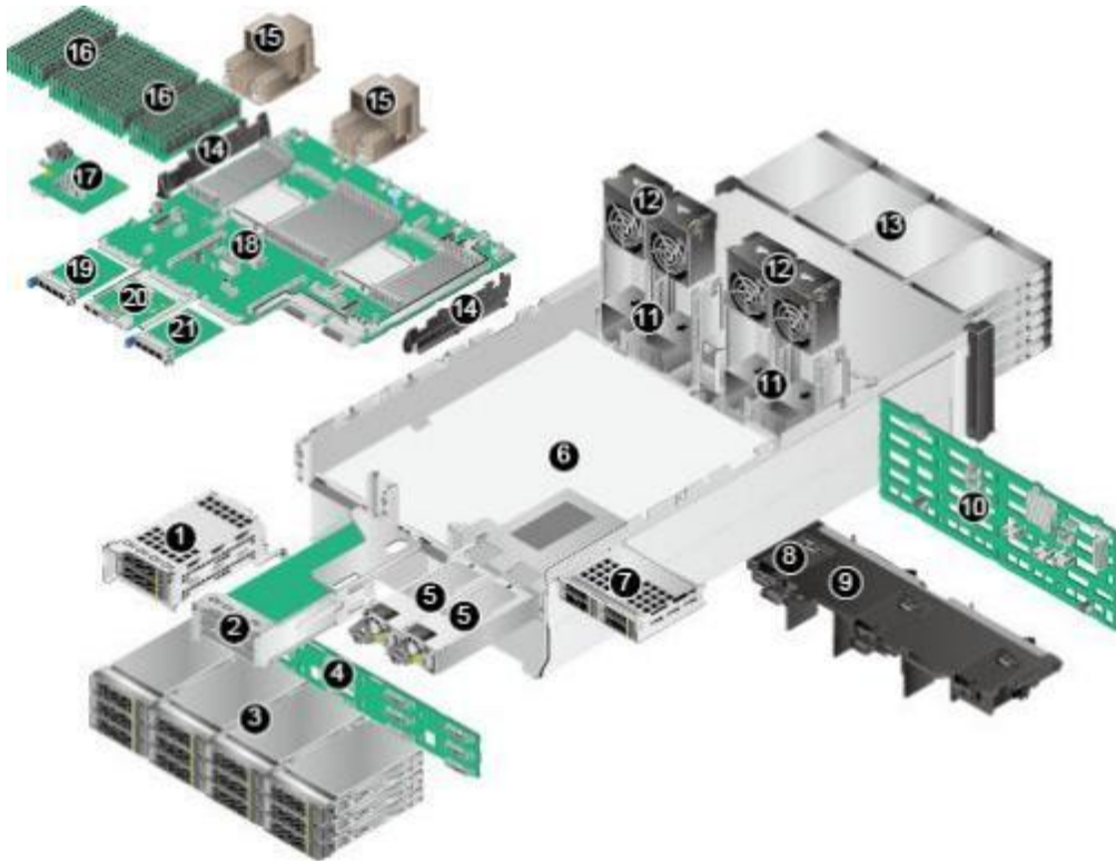
图 4.16：物理结构（配置鲲鹏 920 7260、5250处理器）
