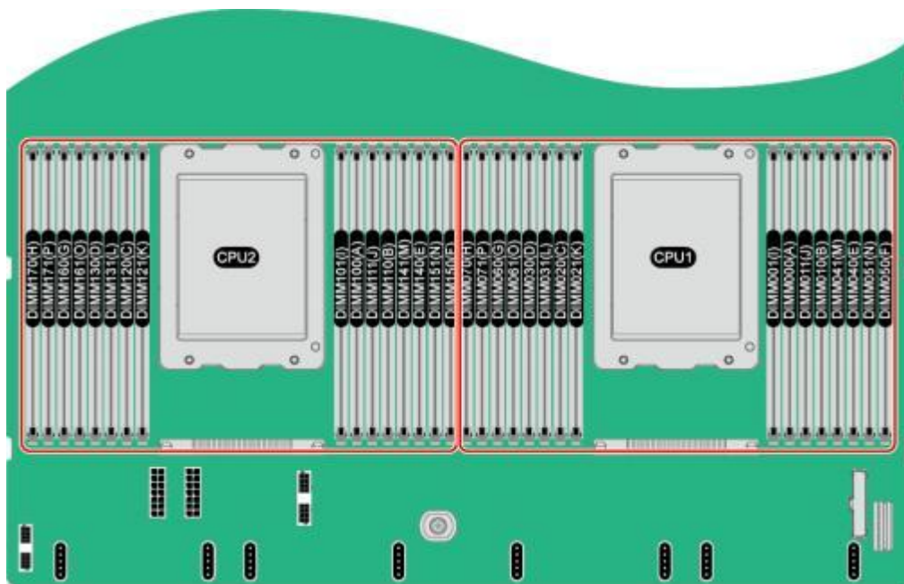
图 6.1: DIMM 安装位置 (鲲鹏 920 7260、5250处理器)
