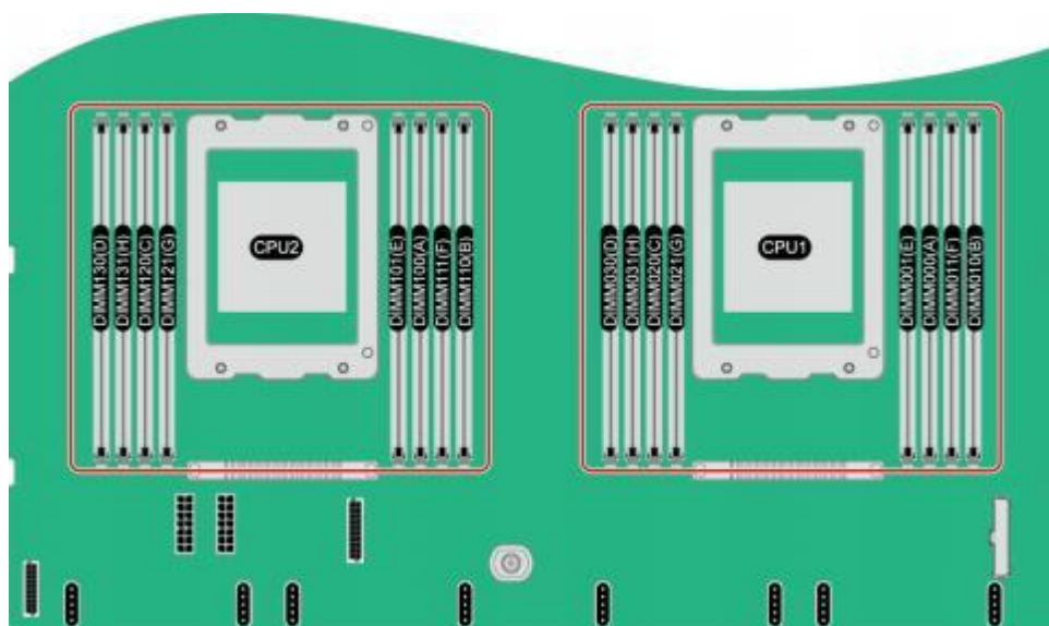
图 6.2、DIMM 安装位置（鲲鹏 920 5220 或 3210 处理器）
