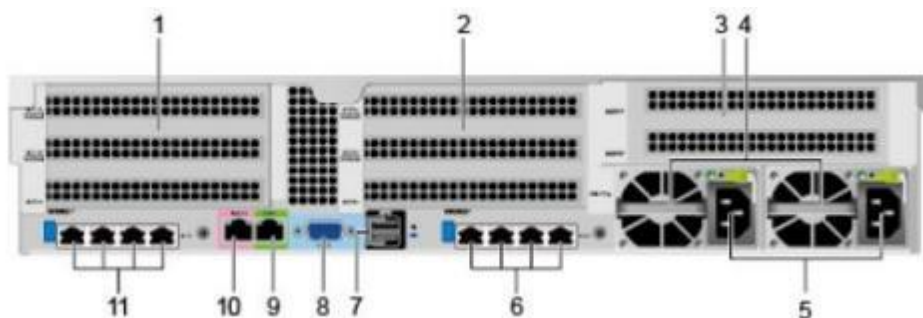
图 4.2：后面板组件
