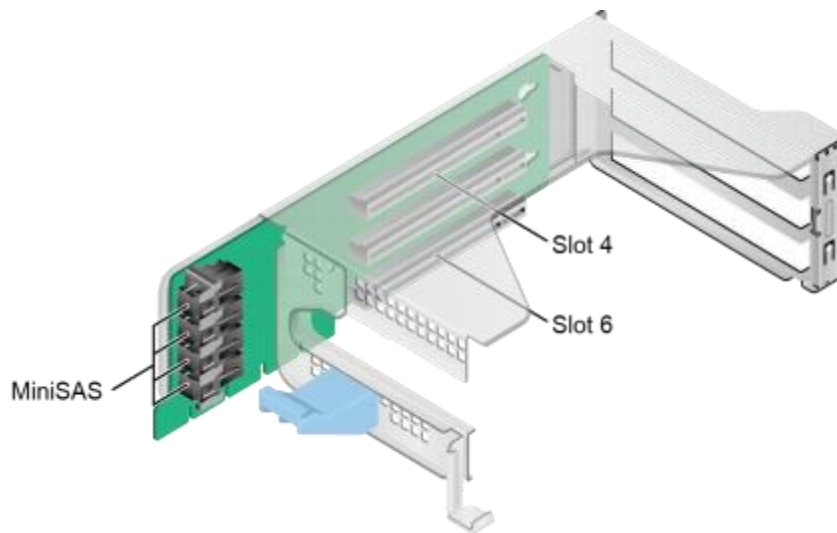
图 4.12: IOB卡 SAS Riser 卡
