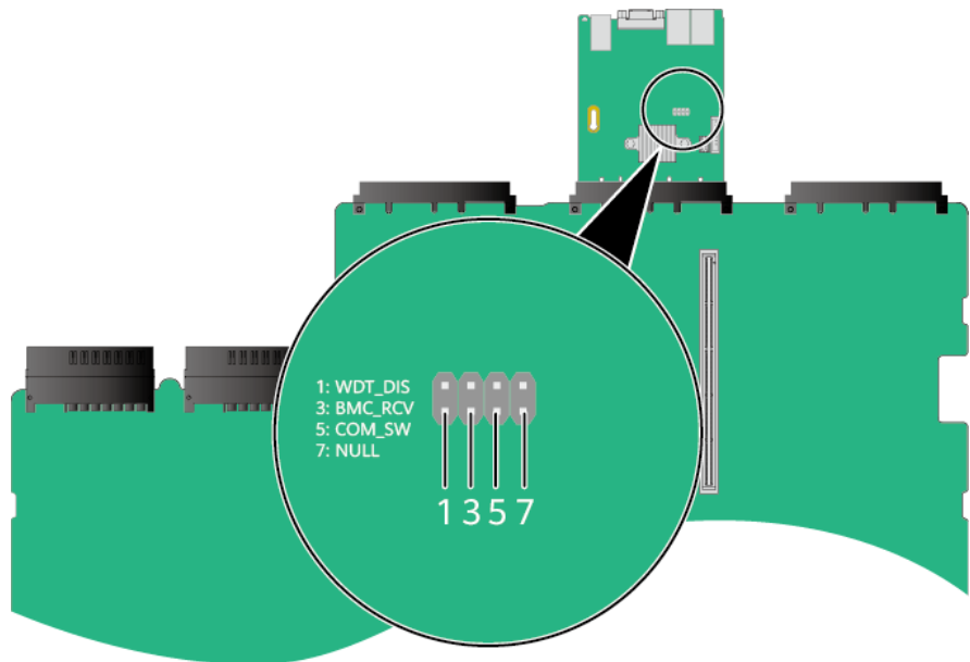
图8-13 跳线位置
