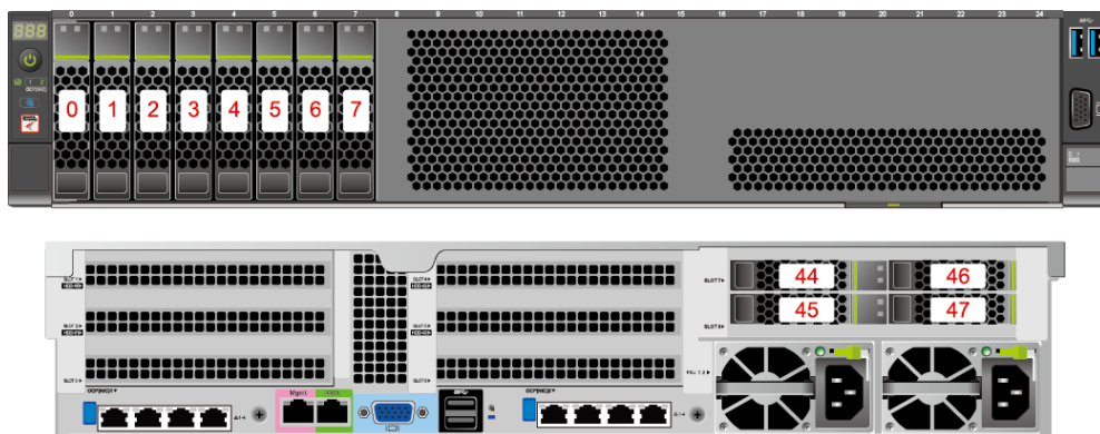
图3-16 8x2.5 英寸硬盘配置的硬盘编号
