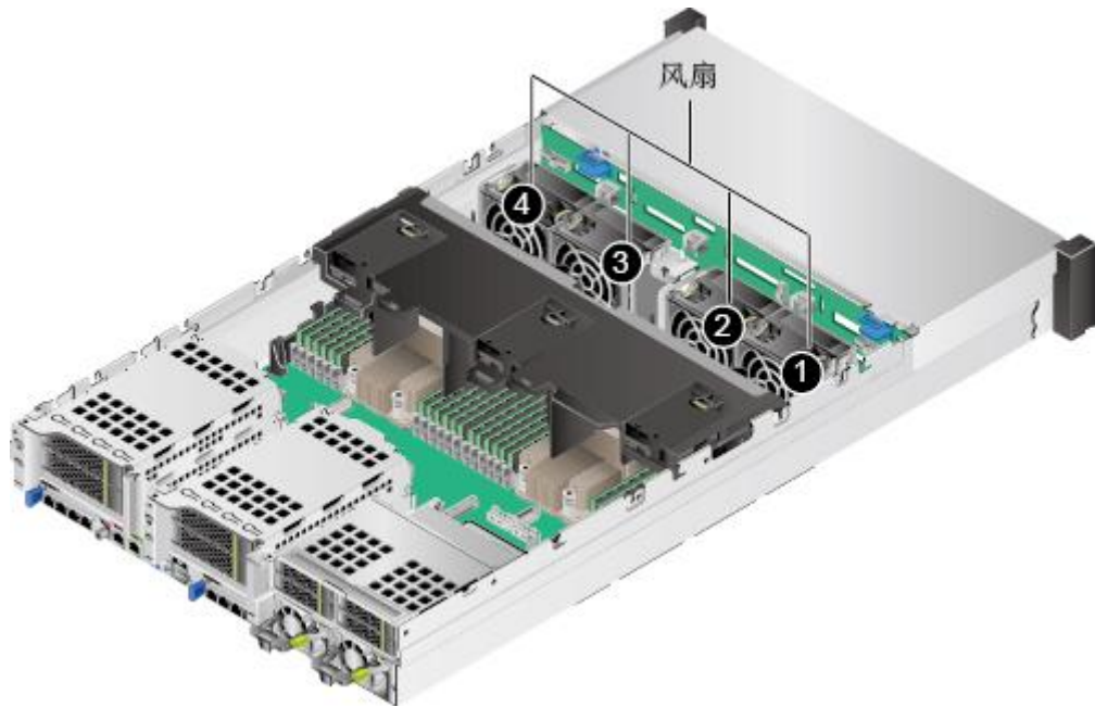
图3-27 风扇位置图
