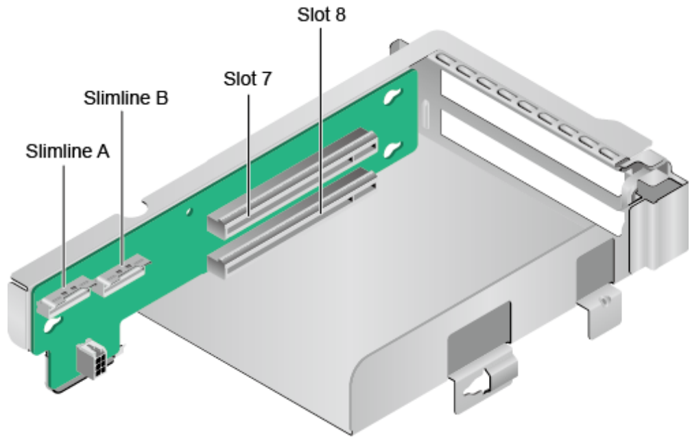
图3-24 Riser 卡 6 (2x8)
