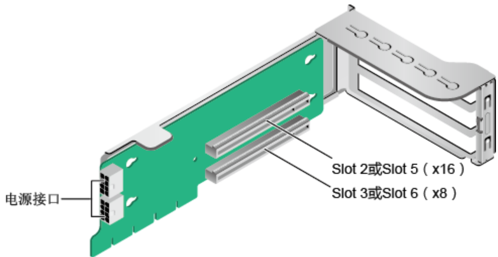
图3-20 Riser 卡 2 (1x8+1x16)
