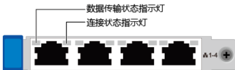
图3-11 TM212（4*GE 电口）
