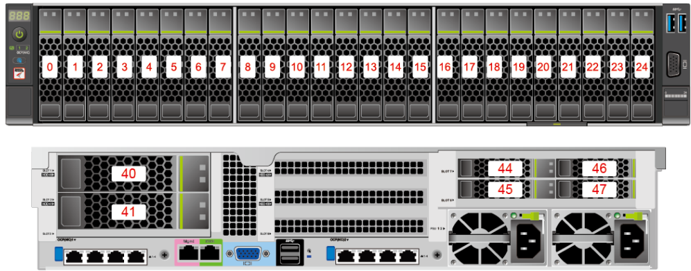
图3-14 25x2.5 英寸硬盘 EXP 配置硬盘编号
