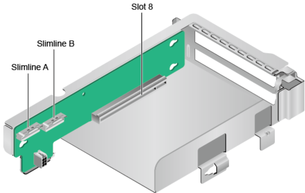
图3-25 Riser 卡 7 (1x16)
