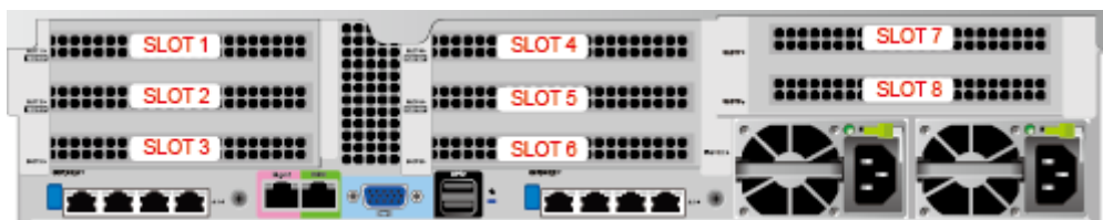
图3-26 PCIe 插槽
