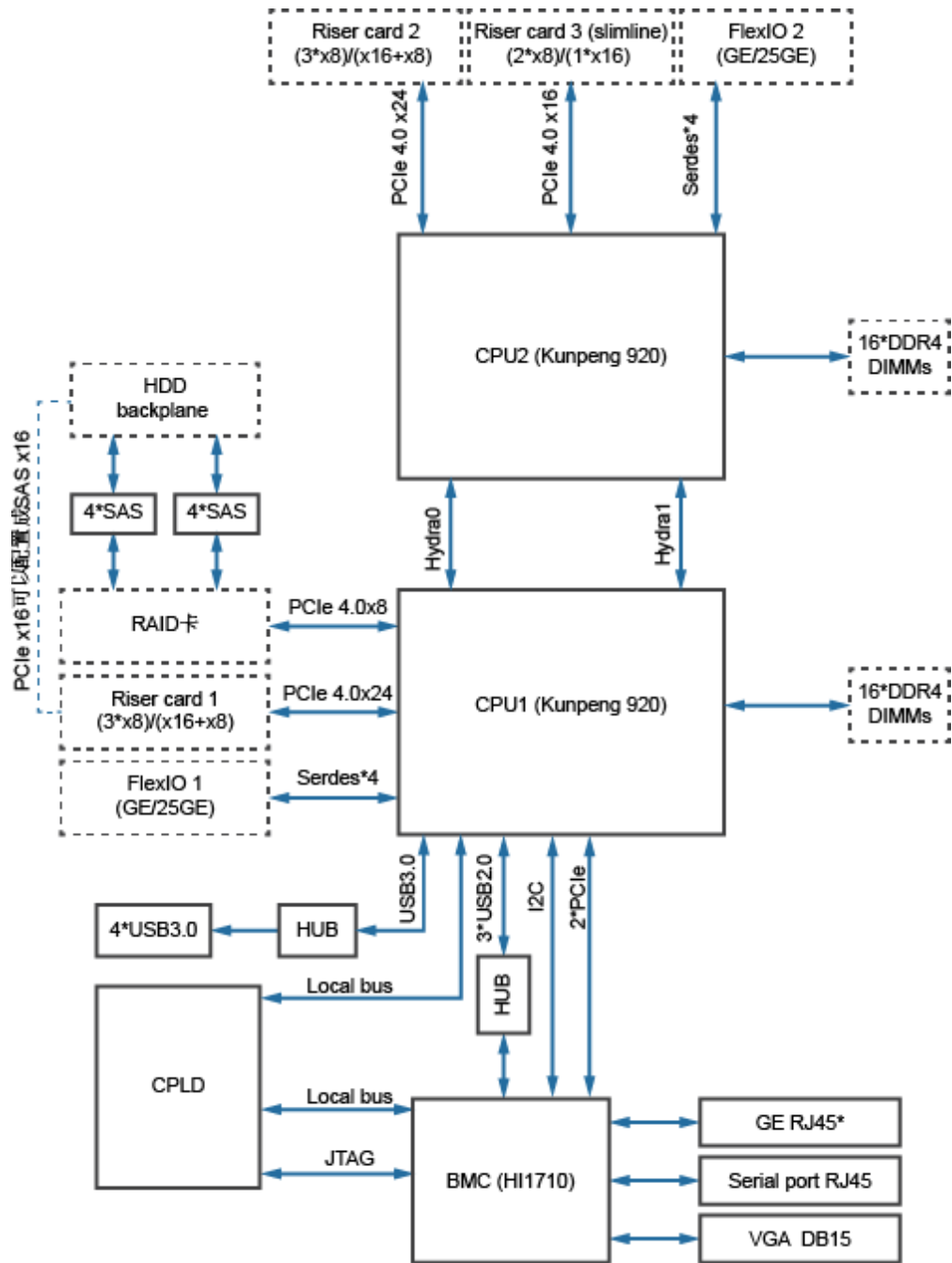
图2-3 逻辑结构
