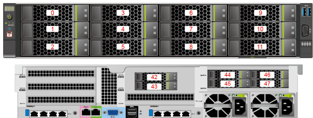
图3-13 12x3.5 英寸硬盘直通配置
