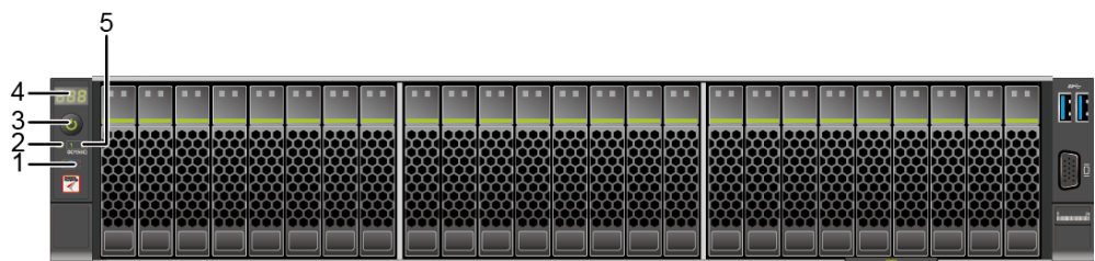
图3-6 25x2.5 英寸硬盘配置前面板指示灯和按钮
