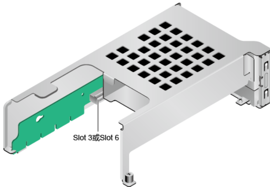
图3-22 Riser 卡 4 (1x16)
