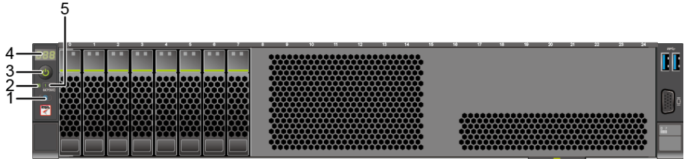
图3-8 8x2.5 英寸硬盘配置前面板指示灯和按钮
