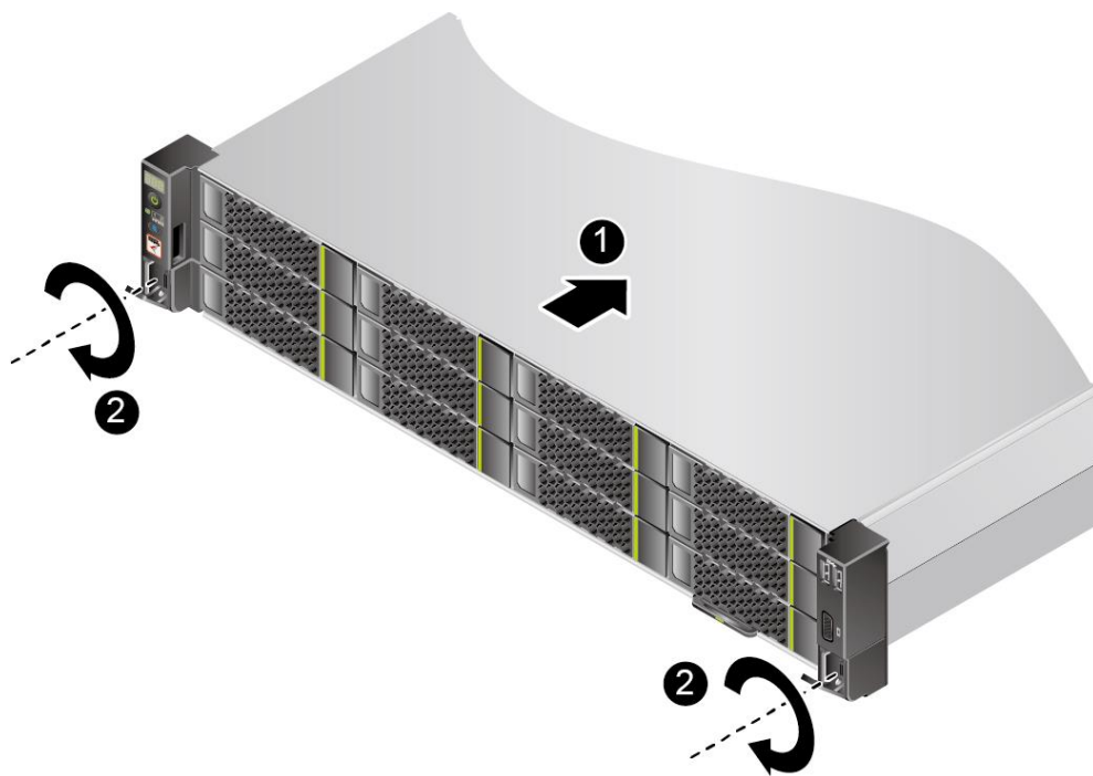
图6-7 安装服务器
