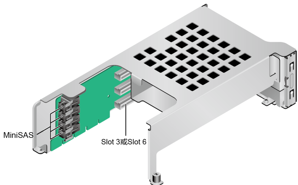
图3-23 Riser 卡 5 (SAS Riser)
