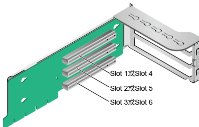
图3-19 Riser 卡 1 (3x8)
