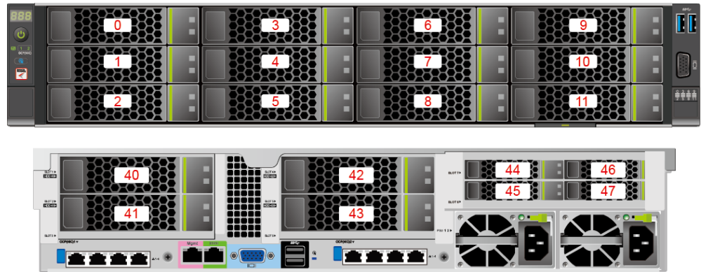
图3-12 12x3.5 英寸硬盘 EXP 配置硬盘编号
