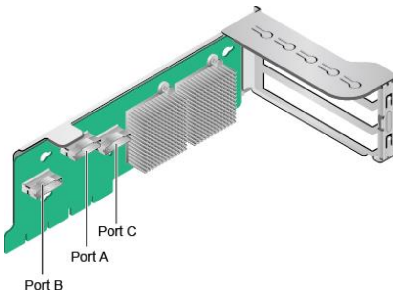
图3-21 Riser 卡 3 (12NVMe 专用)
