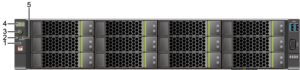
图3-5 12x3.5 英寸硬盘配置前面板指示灯和按钮
