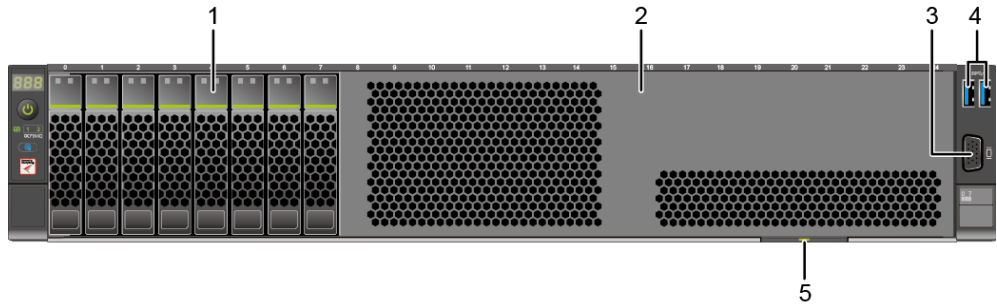
图3-4 8x2.5 英寸硬盘配置前面板组件
