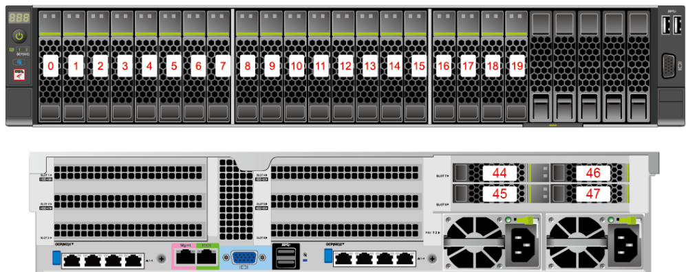
图3-15 8x2.5 SAS/SATA+12x2.5 NVMe 硬盘配置硬盘编号
